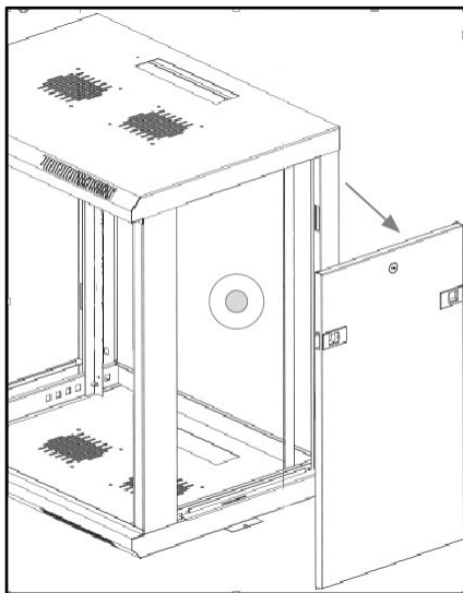
Seitenwand entfernen
