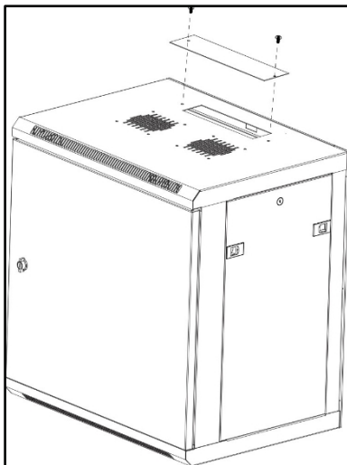
Öffnen der Kabelabdeckung
