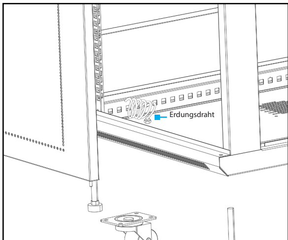
Erdungsdraht
